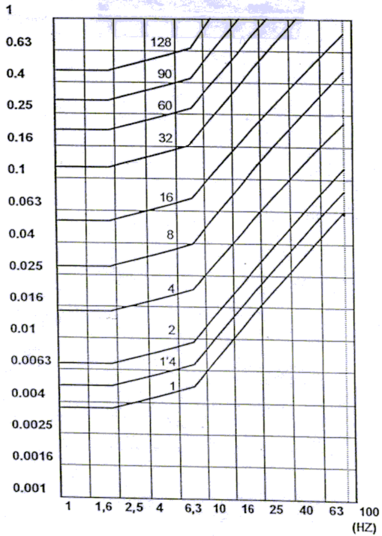
GRÁFICO Nº 1 CURVAS BASES DE NIVELES DE INMISIÓN DE VIBRACIONES
